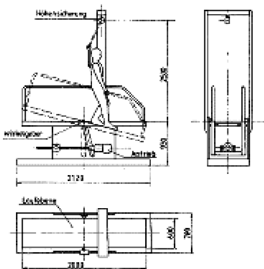
Bild 2: Prüfeinrichtung (Schiefe Ebene)
